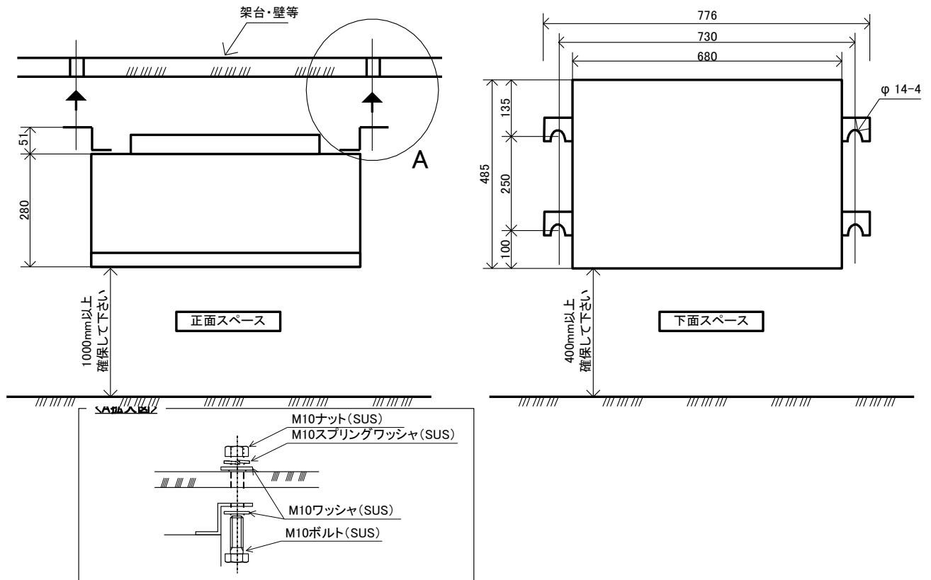
図 2.7 据え付け参考図
