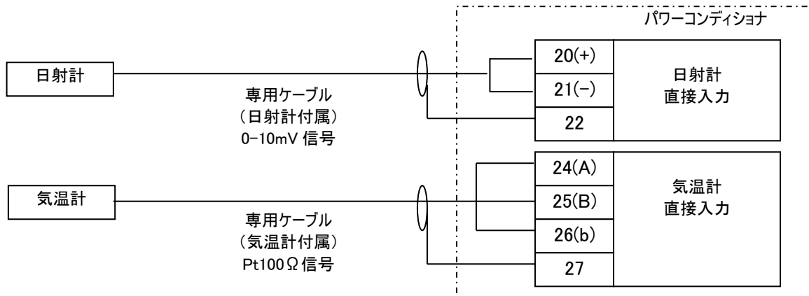
図 6.5.1-1 日射計・気温計を直接入力する場合
