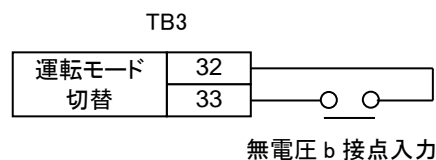
図6.10.1 接続方法例
