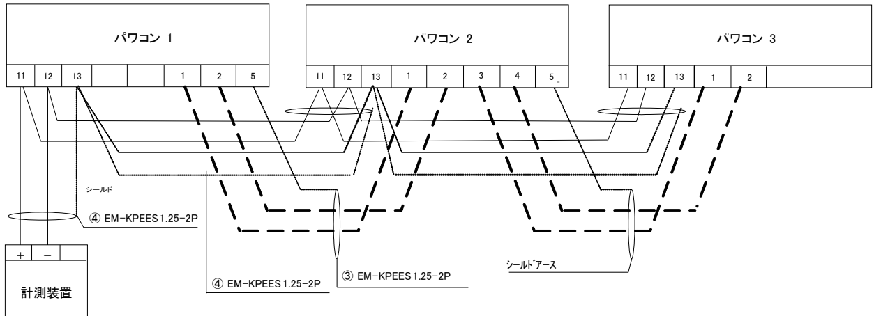
図 6.3 ユニット間の配線例
