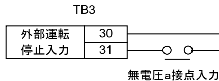
図6.9.1 接続方法例
