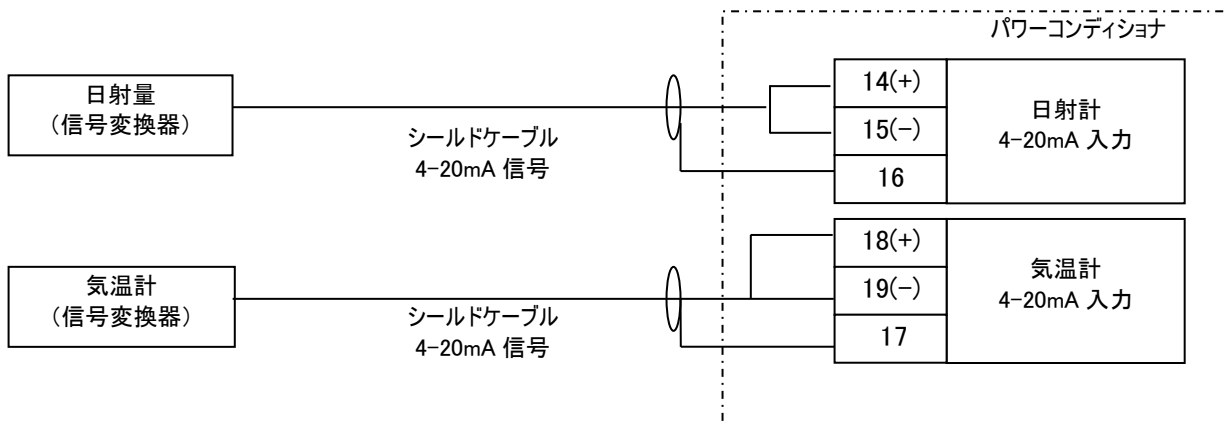
図 6.5.1-2 4-20mA 信号を入力する場合
