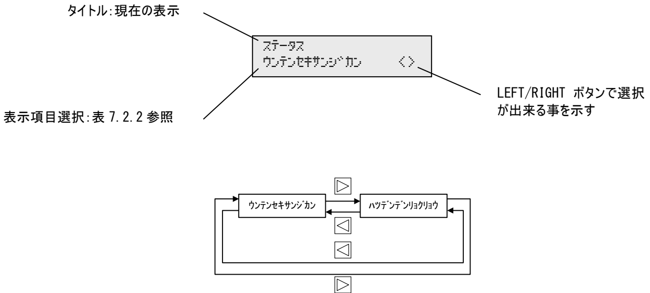
図 7.2.2 ステータス表示順
