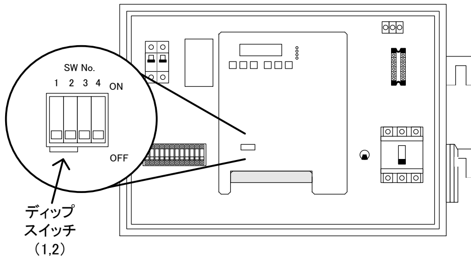
図6.5.2 ディップスイッチの位置
