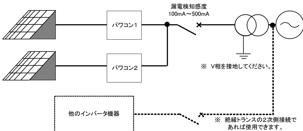
図 6.4.3 系統電源側の配線例 (その他の結線例)
