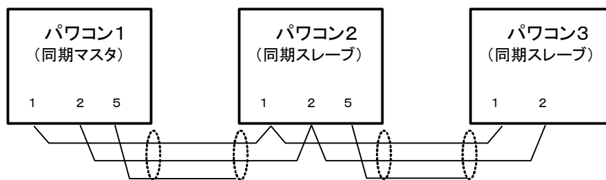
図 6.7.1 パワーコンディショナ3台設置時の接続例
