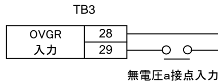
図6.8.1-1 接続方法例
