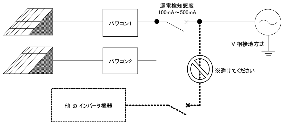
図 6.4.2 系統電源側の配線例 (V 相接地)
