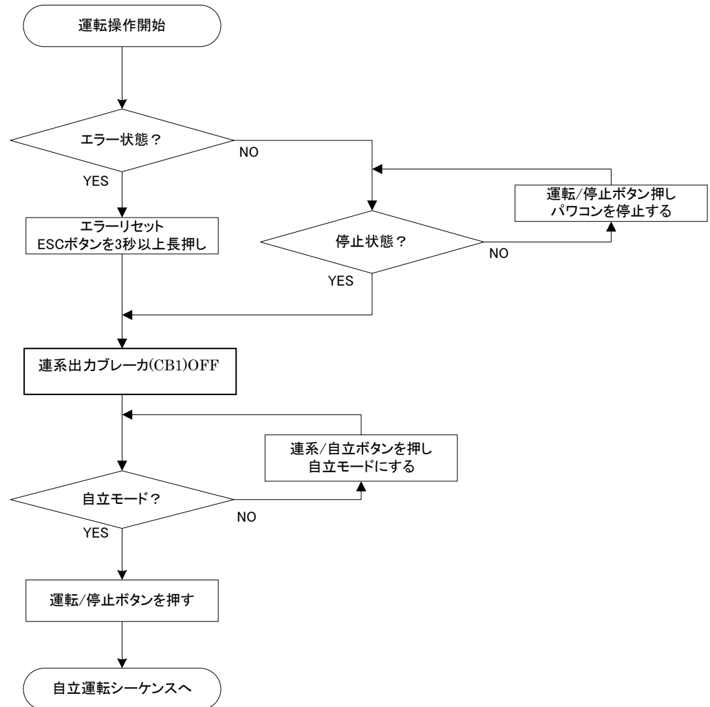
図 7.6.1 自立運転フローチャート
