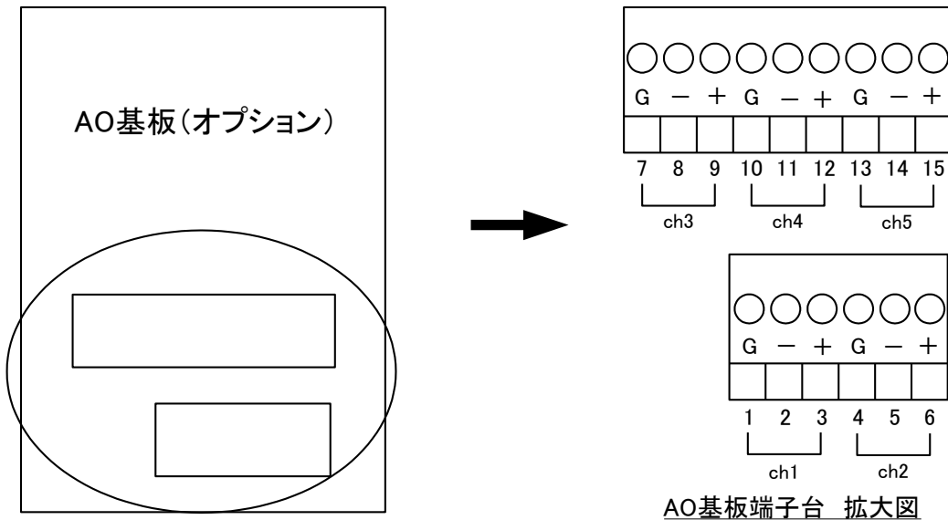
図 6.11 アナログ出力基板端子台配線
