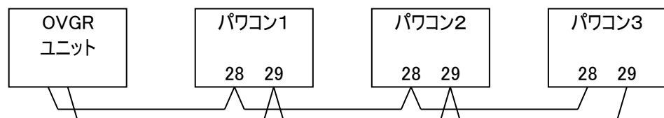
図6.8.1-2 複数台接続例
