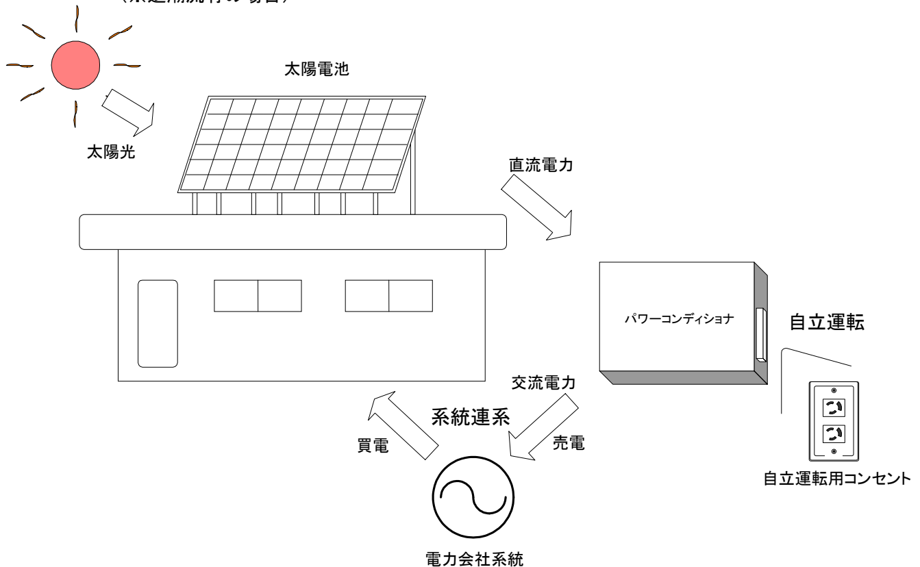
図3 逆潮流有システム例
